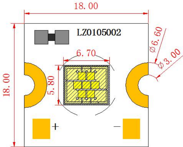
俯视图
