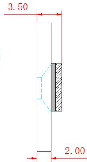
侧视图
